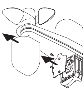
1 - Zdjąć białą dolną osłonę. Otworzyć skrzynkę połączeniową.
