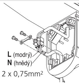
3 - Proveďte zapojení kabelů.
