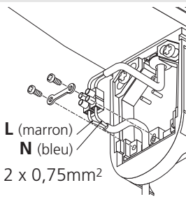
3 - Effectuer le câblage.
