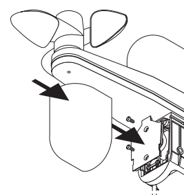
4 - Zamknąć skrzynkę połączeniową.
