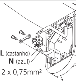
3 - Efectuar as ligações.
