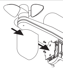
4 - Fermer le boîtier de connexion. Mettre en place le capot blanc et le clipeur
