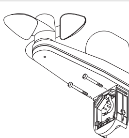
2 - Fixar o automatismo.
