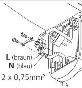
3 - Führen Sie die Anschlüsse aus.
