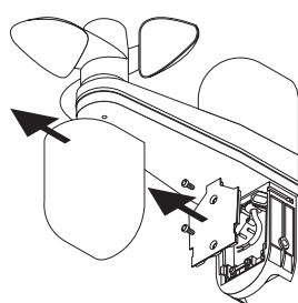
1 - Entfernen Sie die weiße Haube unten. Öffnen Sie das Anschlussgehäuse
