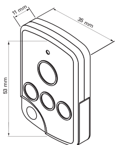
Dimension : 53 x 35 x 11 mm
